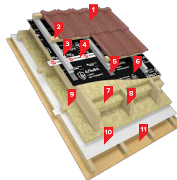
Рис. 6. Строение кровельной системы ТН-ЛЮКСАРД Мансарда
