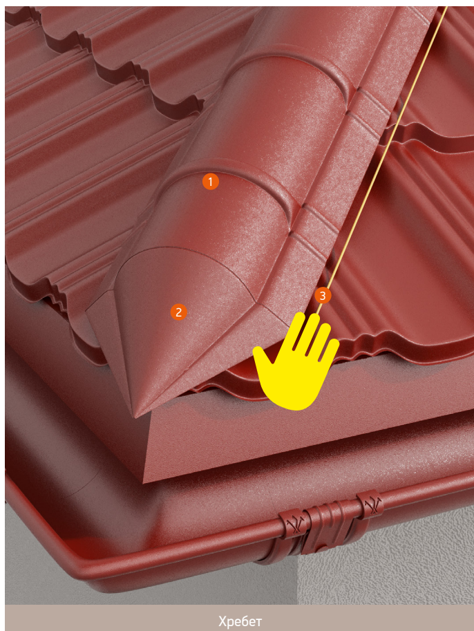
1. Конёк полукруглый
